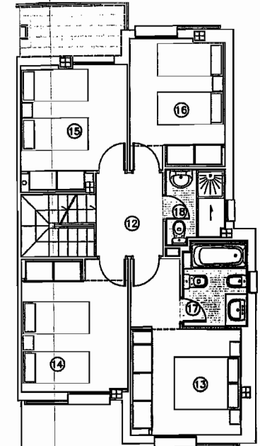
PLANTA PRIMERA
