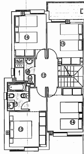
PLANTA PRIMERA
