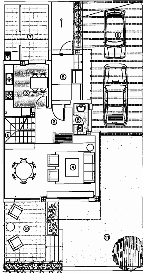
PLANTA BAJA
