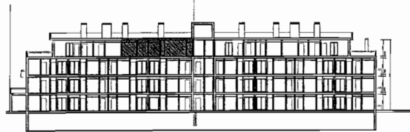
UBICACION DE VIVIENDA A.B EN ALTURA
