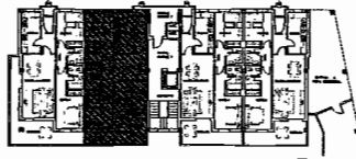
UBICACION DE VIVIENDA B.B EN BLOQUE 1
